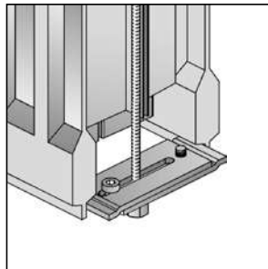
Konternmutter aufdrehen und festschrauben.
